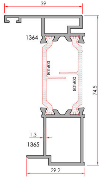
Outward Opening Middle Adapter Dışa Açılır Orta Adaptör
