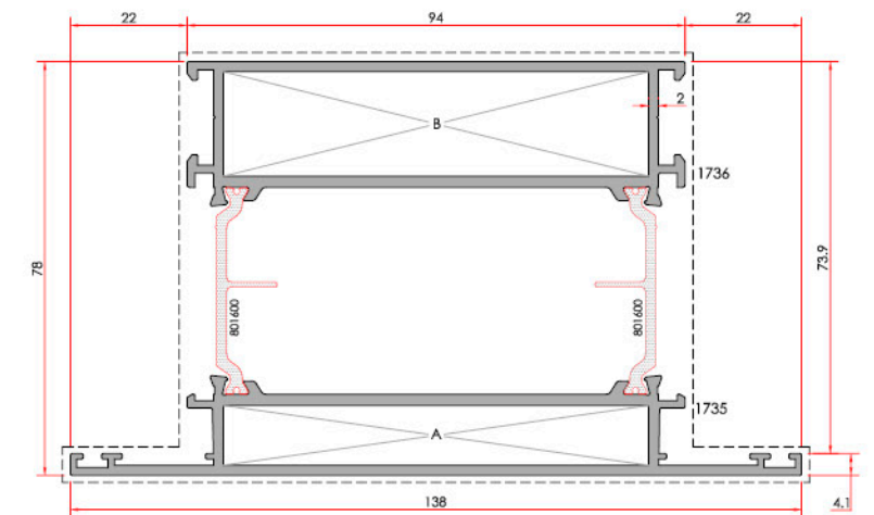
Transom Orta Kayıt
