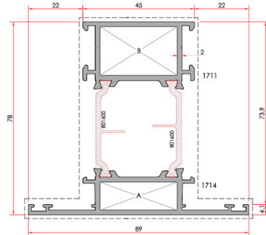
Transom Orta Kayıt
