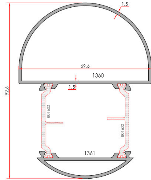
Corner Profile Köşe Dönüş Profili
