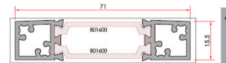
Insulated Sill Profile Yalıtımlı Eşik Profili
