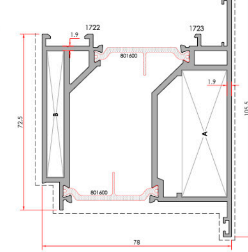
Outward Opening Sash Dışa Açılır Kanat
