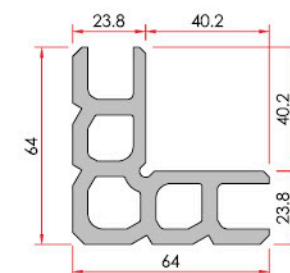
Corner Cleat Köşe Takozu
