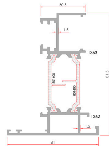
Double Vent Adapter Çift Kanat Adaptörü
