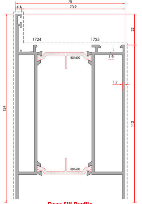
Door Sill Profile Kapı Etek Profili
