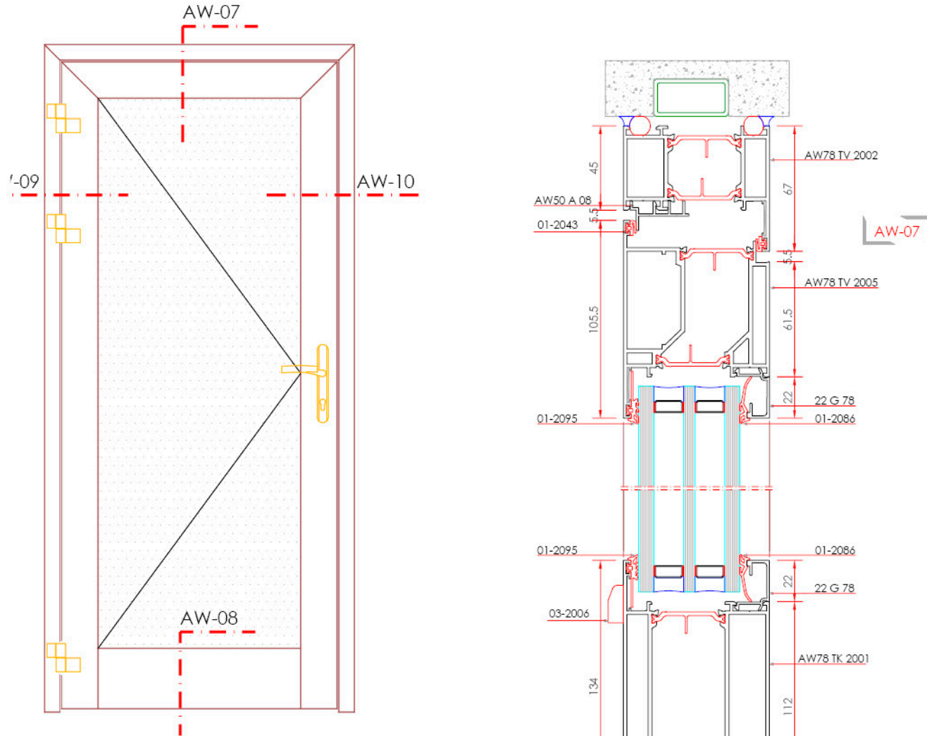
Exterior View - Dış Görünüş
