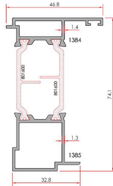
Outward Opening Vent Dışa Açılır Kenar Adaptör
