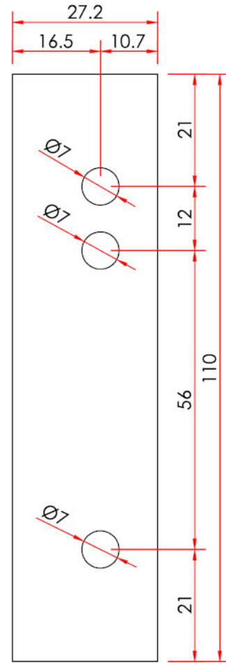
Ölçek:1/1 Ön Görünüş
