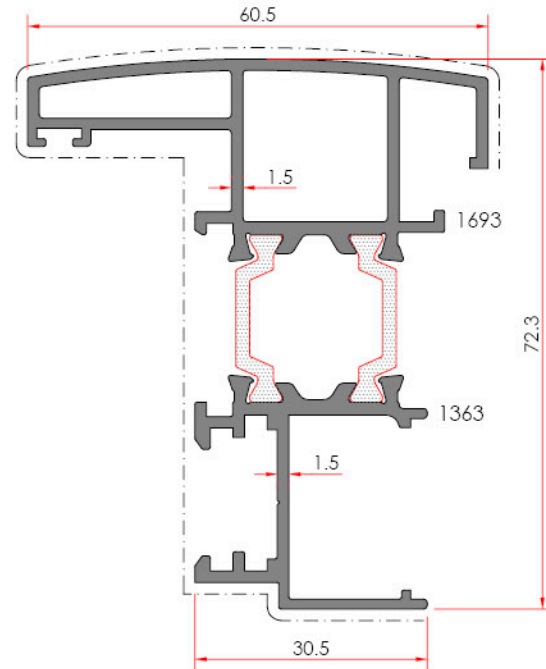
Double Sash Adapter Çift kanat Adaptörü
