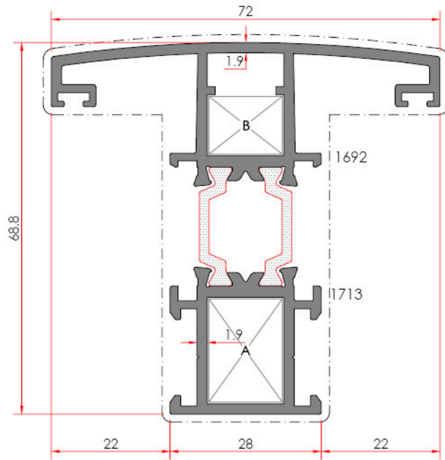
Transom Orta Kayıt
