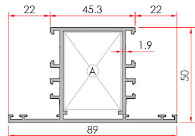
Meeting Rail Orta Kayıt
