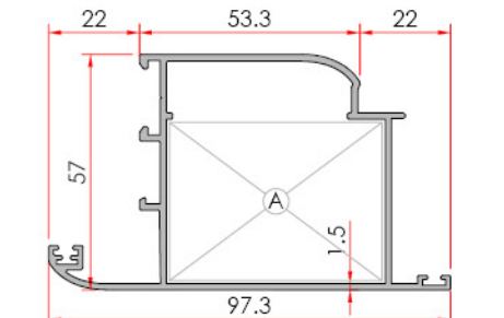
Outward Opening Vent Dışa Açılır Kanat
