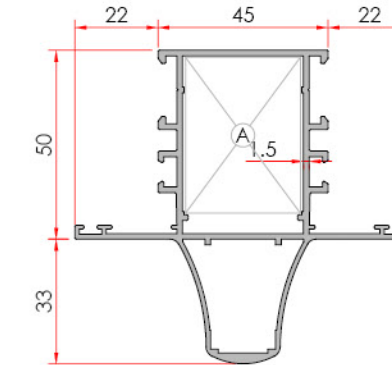
Reinforced Meeting Rail Takviyeli Orta Kayıt
