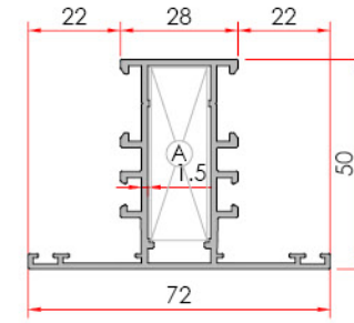
Narrow Meeting Rail Dar Orta Kayıt
