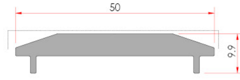
Swing Hinge Bottom Çarpma Menteşe Altı
