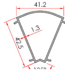
135° Corner Adapter 135° Köşe Dönüş Adaptörü
