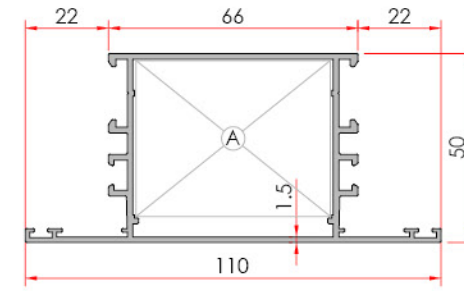
Meeting Rail Geniş Orta Kayıt
