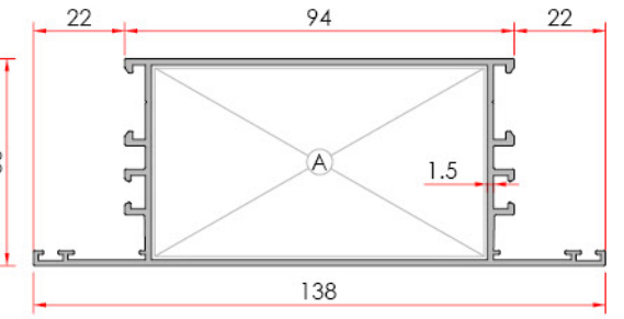
Base Meeting Rail Baza Orta Kayıt
