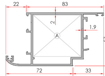
Door Vent Kapı Kanat
