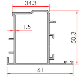
Pivoting Adapter Pivot Adaptörü
