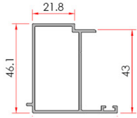
Outward Opening Adapter Dışa Açılır Adaptör
