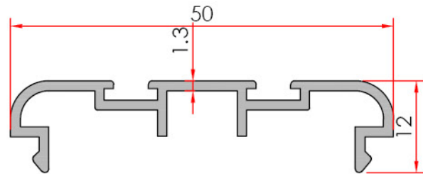
Swing Door Adapter Çarpma Kapı Adaptörü
