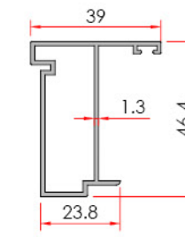
Outward Opening Middle Adapter Dışa Açılır Orta Adaptörü
