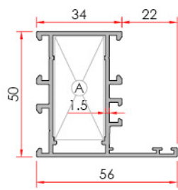
Wide Frame Geniş Kasa
