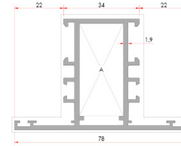
Narrow Transom Dar Orta Kayıt
