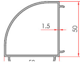
90° Corner Adapter 90° Köşe Dönüş Adaptörü
