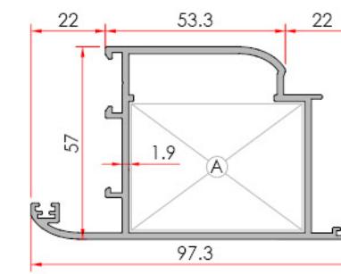
Outward Opening Vent Dışa Açılır Kanat
