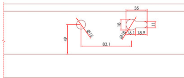
Görünüş -1 Elevation -1 Kol ve Barel İşlemi Handle And Security Cylinder Operation
