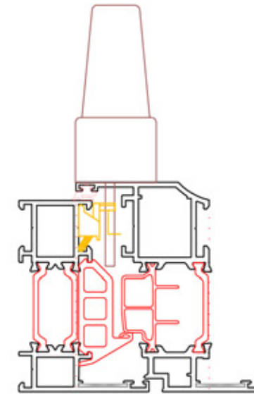
Çift Eksen Açılım Kol Yeri İşlemi Double the axis Arm Part Opening operation
