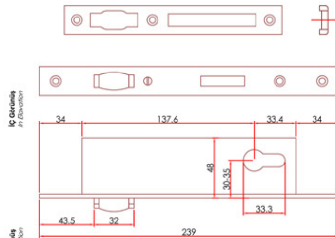
Makaralı Dİİİ Kapı Kilitli Görünüşü Lock Roller Striker Elevation
