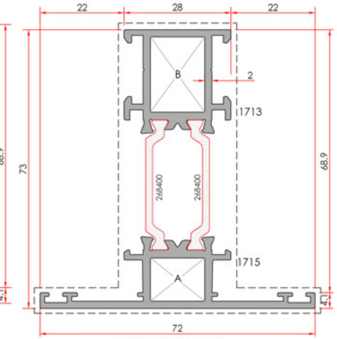
Narrow Meeting Rail Dar Orta Kayıt
