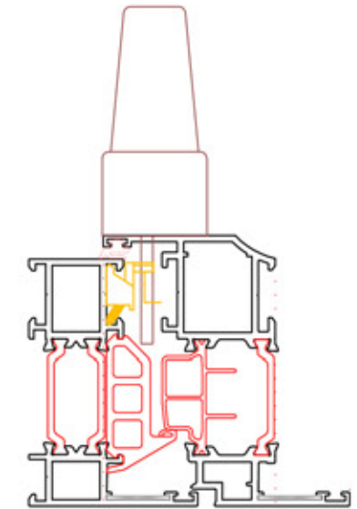
Tek Eksen Sol Açılım Kol Yeri İşlemi Single the axis Opening Left Arm Part operation
