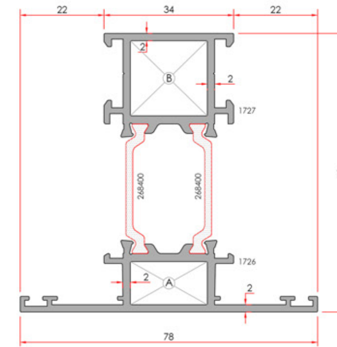
Meeting Rail Orta Kayıt
