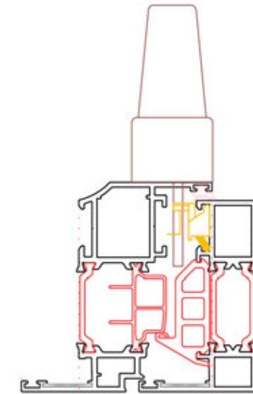
Tek Eksen Sağ Açılım Kol Yeri İşlemi Single the axis Opening Right Arm Part operation
