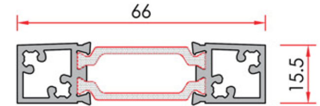
Insulated Sill Profile Yalıtımlı Eşik Profili
