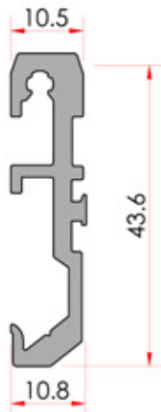
Meeting Rail Connection Orta Kayıt Bağlantı
