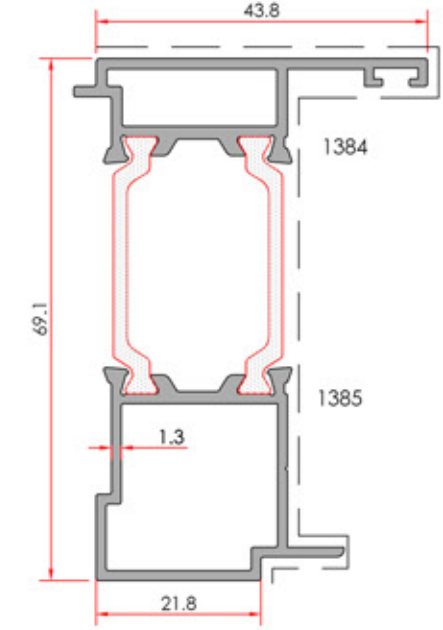
Outward Opening Adapter Dışa Açılır Kenar Adaptör
