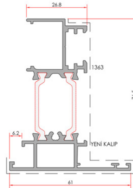
Double Sash Adapter Çift Kanat Adaptörü
