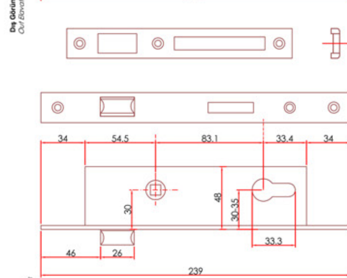
Düzi Kapı Kildi Görünüşü Lock Striker Elevation
