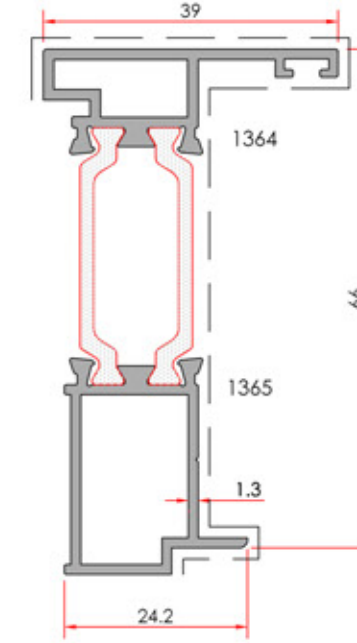
Outward Opening Middle Adapter Dışa Açılır Orta Adaptör
