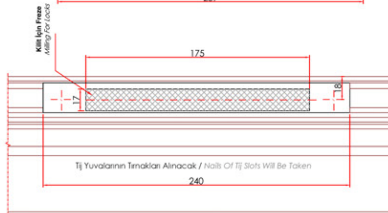
Görünüş -2 Elevation-2 Kapı Kilitli İşlemi Security Door Lock Operation
