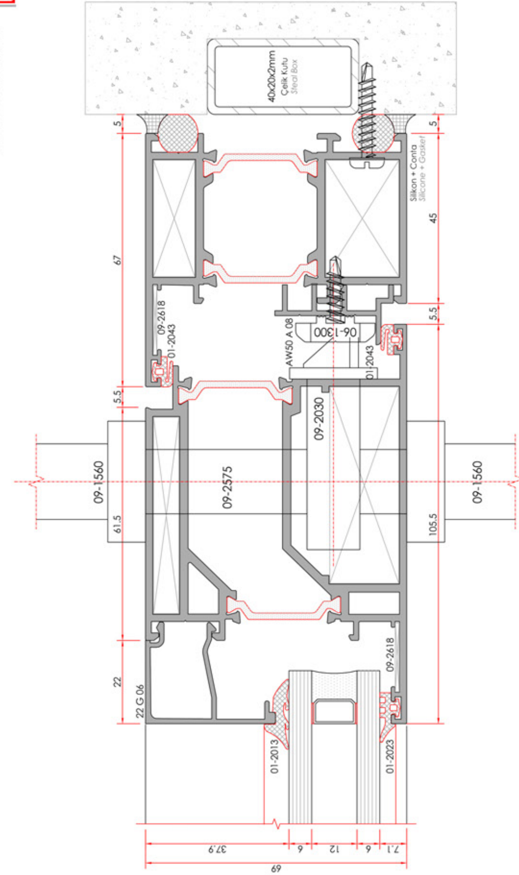
Dış Açılır Sistem Outside Opening System
