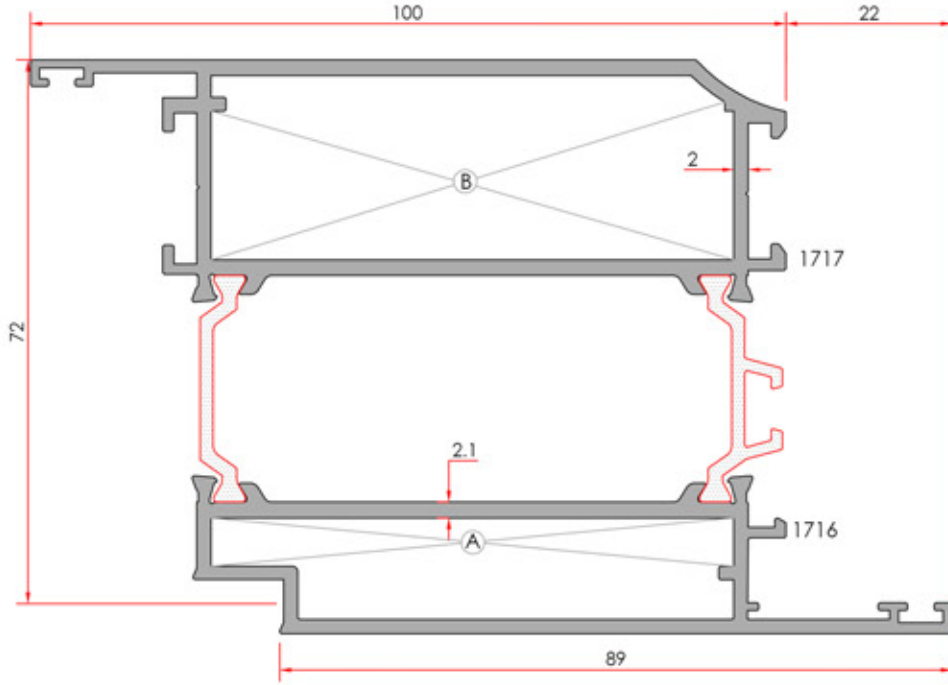
Door Vent Profile Geniş Kapı Kanat Profili
