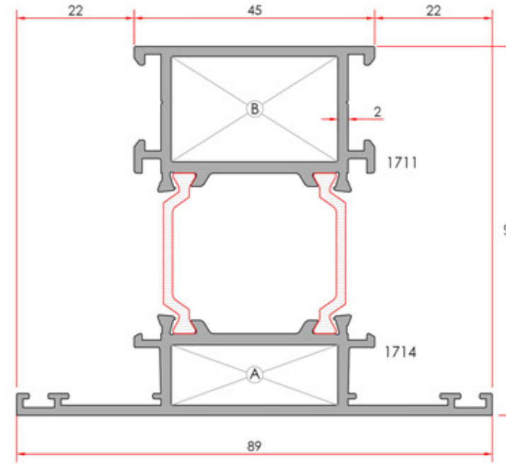
Meeting Rail Orta Kayıt
