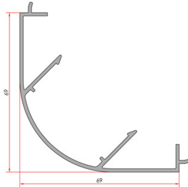
90° Corner Profile (Exterior) 90° Köşe Dönüş Profili (Dış)
