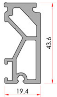
Meeting Rail Connection Orta Kayıt Bağlantı
