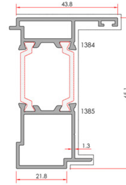
Outward Opening Adapter Dışa Açılır Kenar Adaptör
