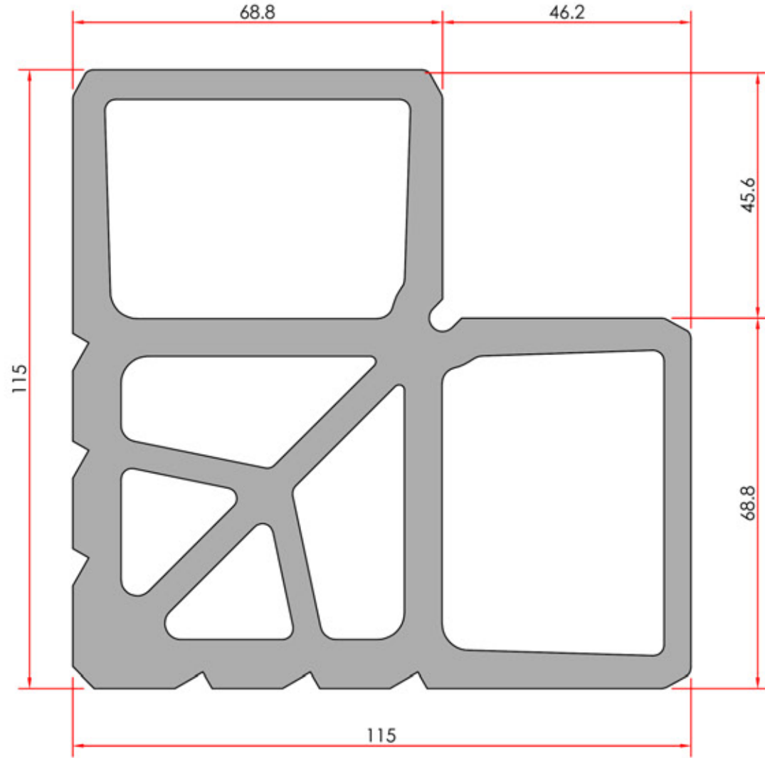
Corner Cleat Köşe Talozu
