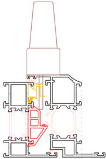
Çift Eksen Açılım Kol Yeri İşlemi Double the axis Arm Part Opening operation
