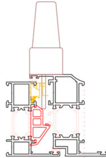
Tek Eksen Sol Açılım Kol Yeri İşlemi Single the axis Opening Left Arm Part operation
