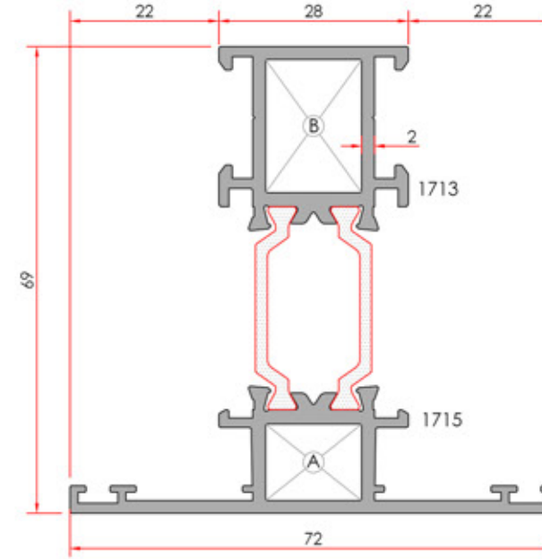
Narrow Meeting Rail Dar Orta Kayıt
