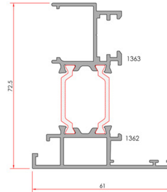
Double Vent Adapter Çift Kanat Adaptörü
