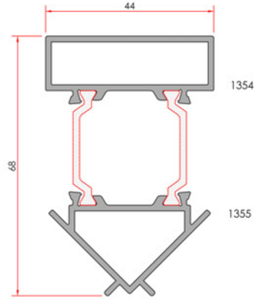
90° Corner Profile (Interior) 90° Köşe Dönüş Profili (İç)
