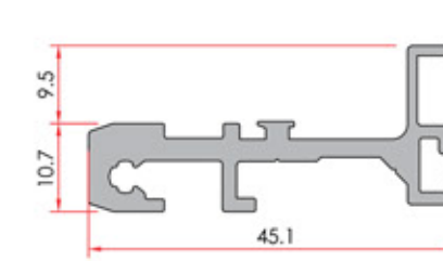
Meeting Rail Connection Orta Kayıt Bağlantı
