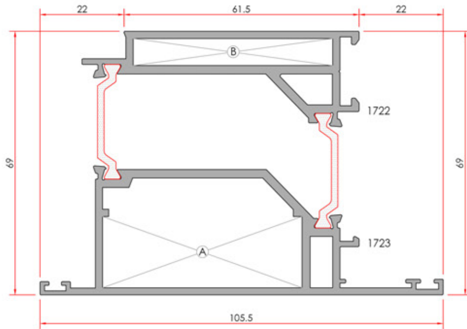
Outward Opening Vent Profile Dışa Açılır Kanat Profili
