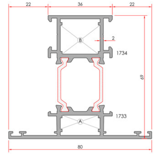
Meeting Rail Orta Kayıt
