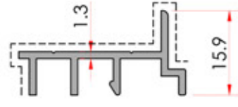
Outward Opening Fixed Adapter Dış Açılır Sabit Adaptör
