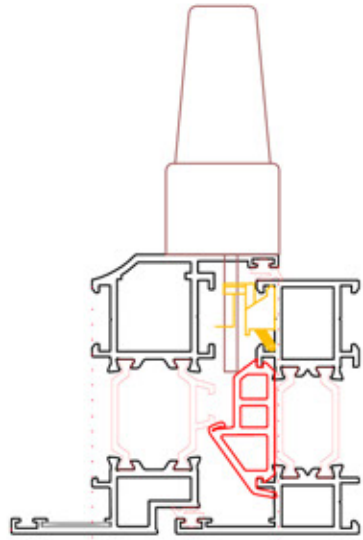
Tek Eksen Sağ Açılım Kol Yeri İşlemi Single the axis Opening Right Arm Part operation
