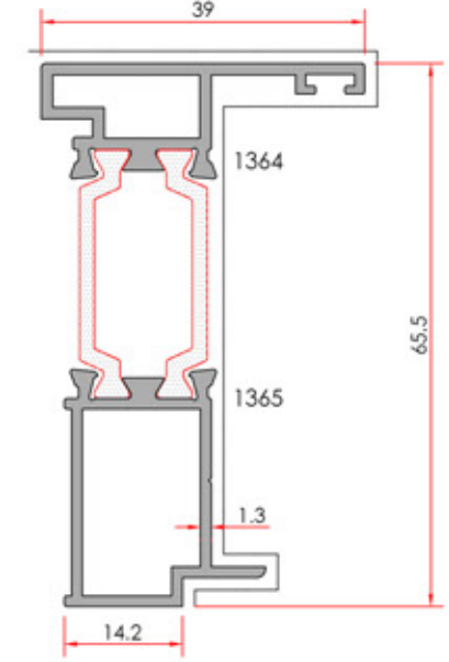
Outward Opening Middle Adapter Dışa Açılır Orta Adaptör
