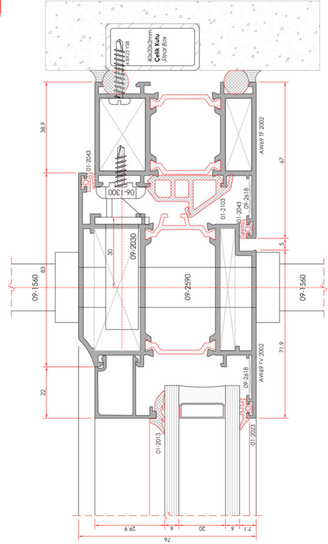
İçe Açılır Sistem Inside Opening System
