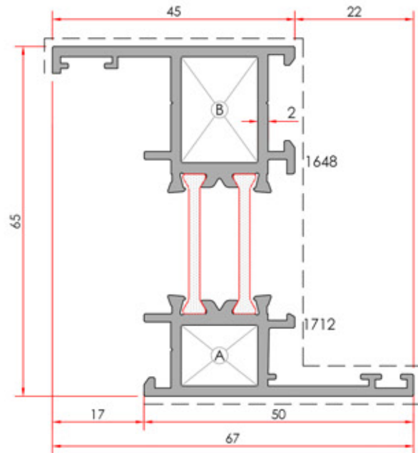
Sill Frame Pervaz Kasa
