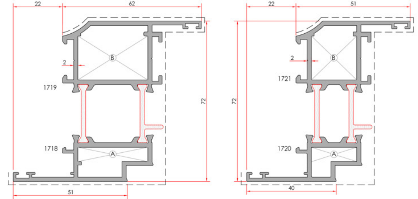
Vent Profile Pencere Kanat Profili
