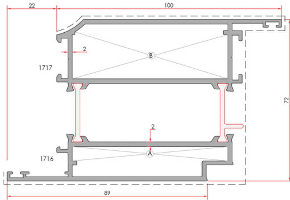
Door Vent Geniş Kapı Kanat Profili
