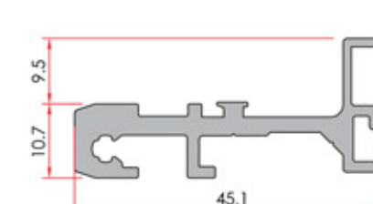
Meeting Rail Connection Orta Kayıt Bağlantı
