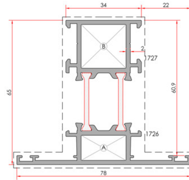
Meeting Rail Orta Kayıt
