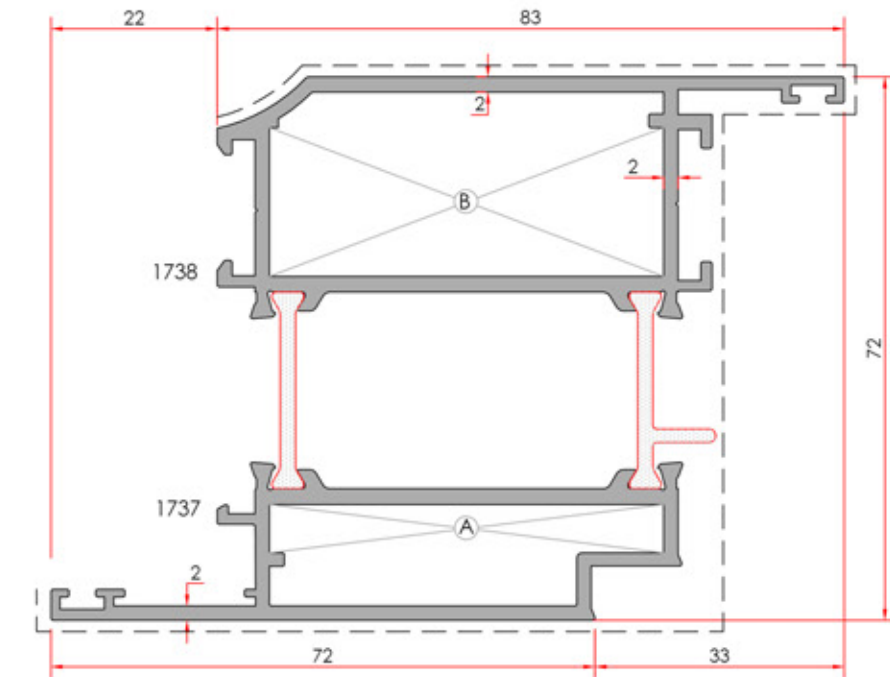
Door Vent Kapı Kanat Profili
