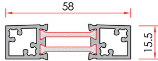
Sill Profile Yalıtımlı Eşik Profili
