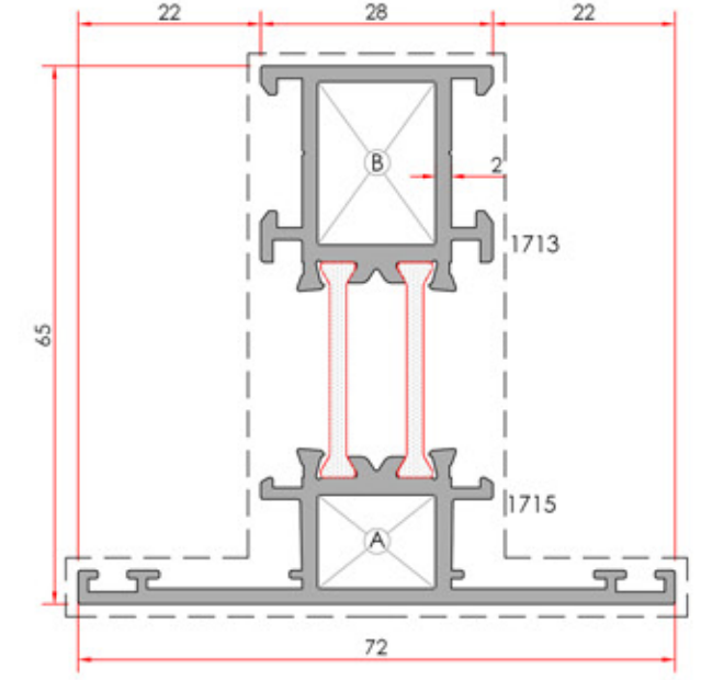
Narrow Meeting Rail Dar Orta Kayıt
