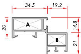
Narrow Glass Panel (Vent) Dar Cam Paneli (Kanat)
