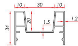
Cover Fugalı Kapak
