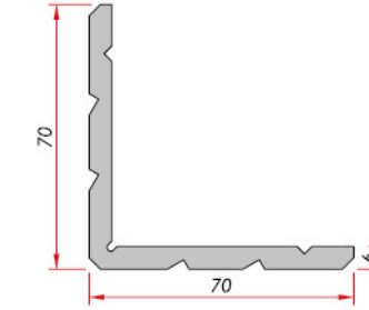
Corner Cleat Köşe Takozu
