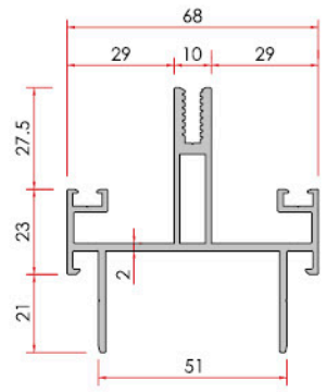
Mullion Mulyon
