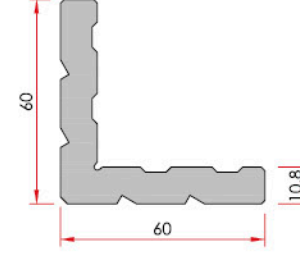
Corner Cleat Köşe Takozu
