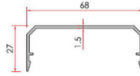
Vertical Cover Düşey Kapak
