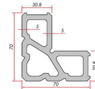
Corner Cleat Köşe Takozu
