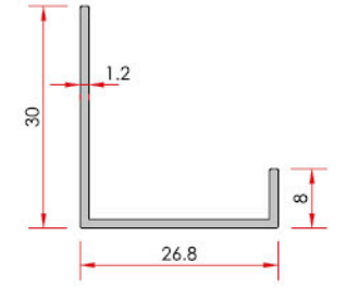
Dilatation Profile Dilatasyon Profili
