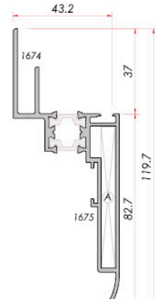
Skylight Vent Işıklı Kanat
