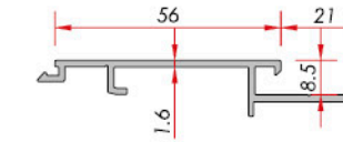
Valve Adapter Kapak Adaptörü
