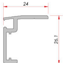
Skylight Vent Adapter Işıklı Kanat Adaptörü
