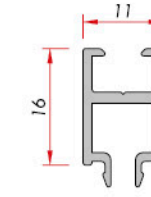
Single Glass Bead Tek Cam Çıtası
