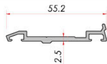
Single Glass Bead Tek Cam Çıtası
