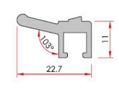
Angle Clips Açılı Klips
