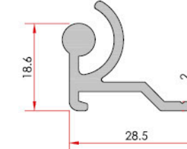
Corner Köşe Dönüş Dış
