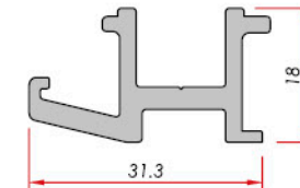
Panel Assembling Wedge Kaset Montaj Takozu
