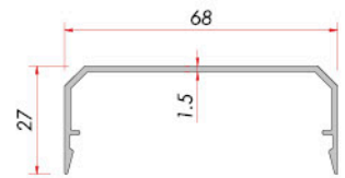
Vertical Cover Düşey Kapak
