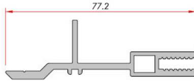
Half Mullion Adapter Yarım Mulyon Adaptörü
