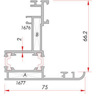
Skylight Frame Işıklı Kasa
