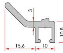
Ext. Corner Turning Clips Dış Köşe Dönüş Klipsi
