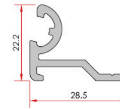
Corner Köşe Dönüş İç
