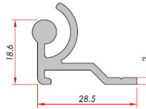
Corner Köşe Dönüş İç
