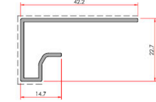
Dilatation Profile Dilatasyon Profili
