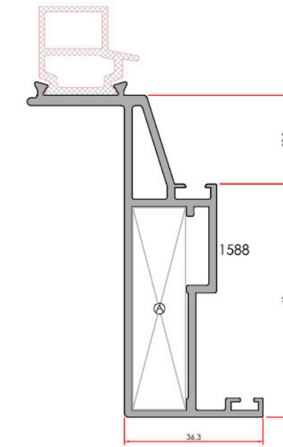
Hidden Wing Frame Gizli Kanat Kasa
