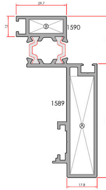
Thermo Vent Yalıtımlı Kanat
