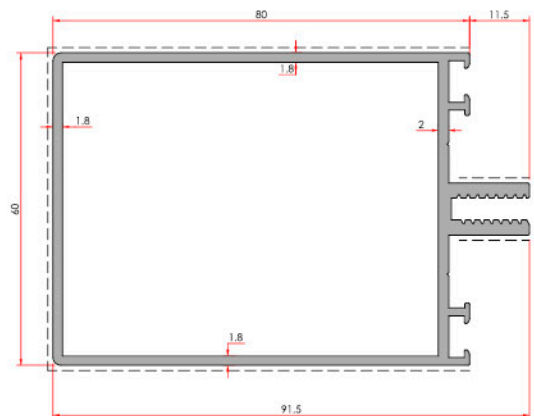
Transom Yatay
