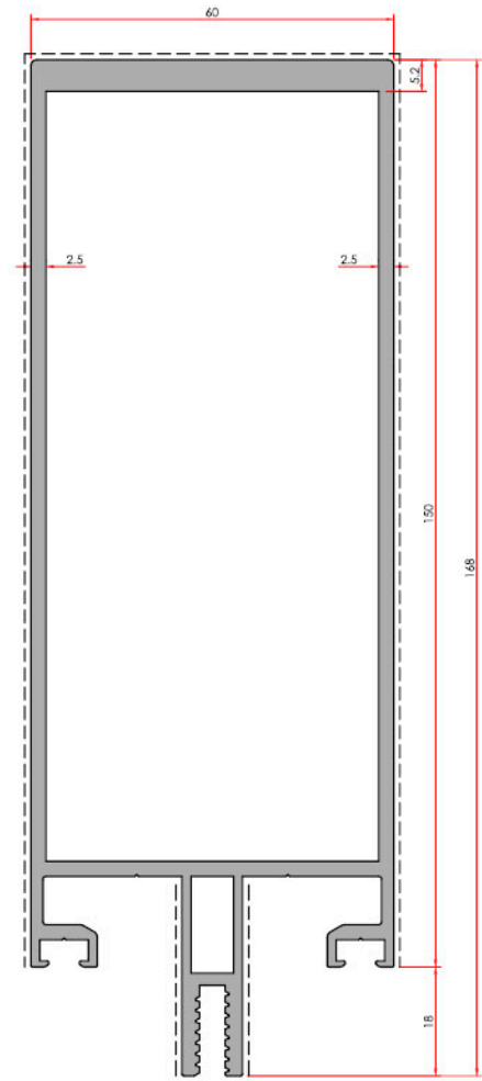
Mullion Düşey
