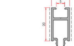
Single Glass Bead Tek Cam Çıtası
