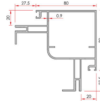
90° Corner Profile 90° Köşe Profili
