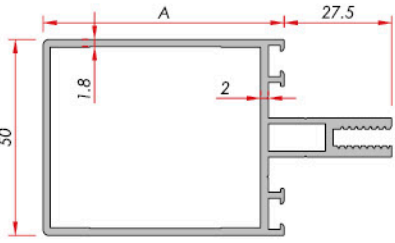
Transom Profiles Transom Profilleri
