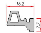
Panel Assembling Clips Kaset montaj Klipsi
