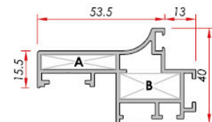
Glazing Panel (Vent) Cam Paneli (Kanat)
