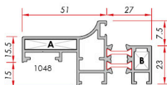
Narrow Glass Panel (Vent) Dar Cam Paneli (Kanat)
