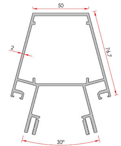
135° Corner Profile 135° Köşe Profili
