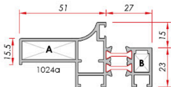
Insulated Glazing Panel (Sash) Yalıtımlı Cam Paneli (Kanat)
